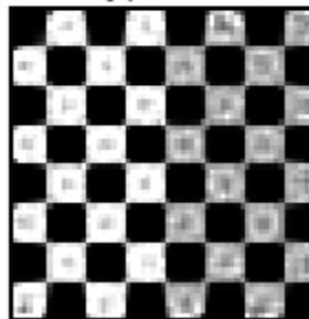
deconvlucy(A,PSF,NI,DP,WT)
