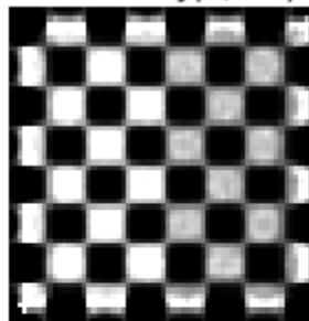
deconvlucy(A,PSF)
